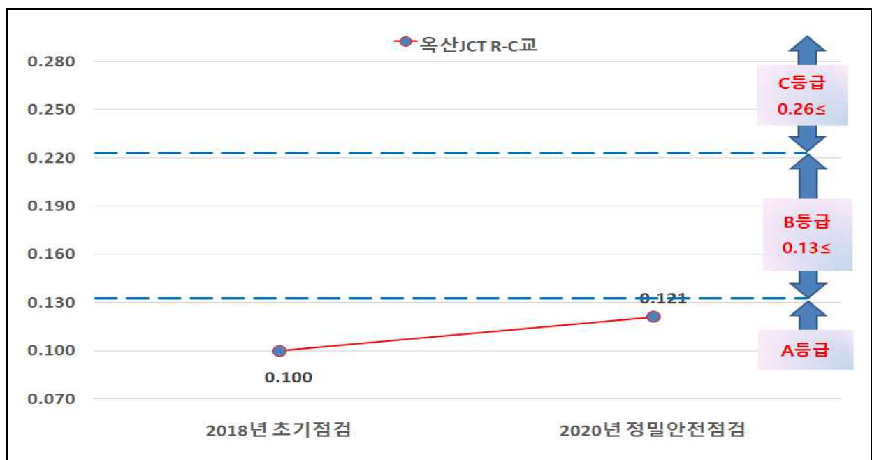
[그림 2.4.1] 옥산JCT RAMP-C교 상태평가 결과 비교 그래프
